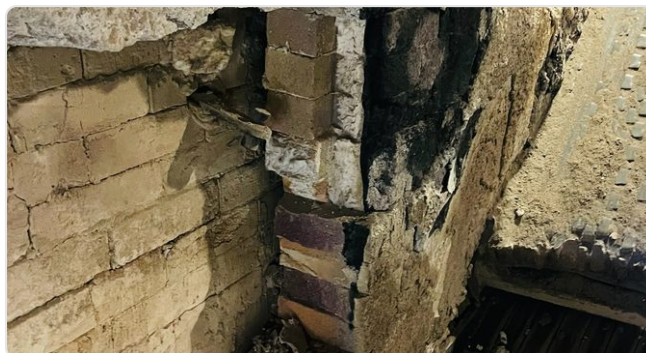
Fisură la trecerea de la zidărie la masa monolitică — se observă
