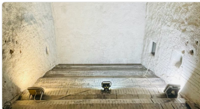
Wyłożenie komory spalania podczas planowanego postoju
